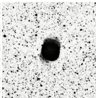
NGC6781 P.N. 10.0'
