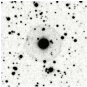
NGC6826 P.N. 5.0'
