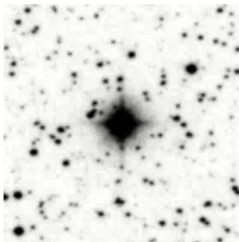
NGC6572 P.N. 4.0'
