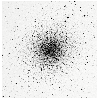
NGC5897 G.C. 15'
