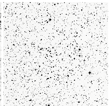
NGC 6811 O.C. 20.0'
