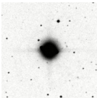
NGC7009 P.N. 5.0'
