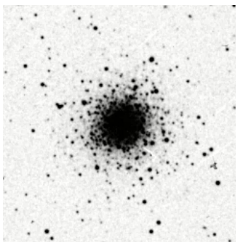
NGC 6229 G.C. 7.0'
