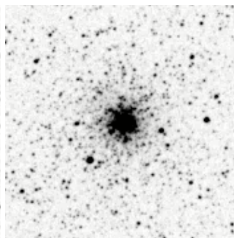
NGC6316 G.C. 5.0'
