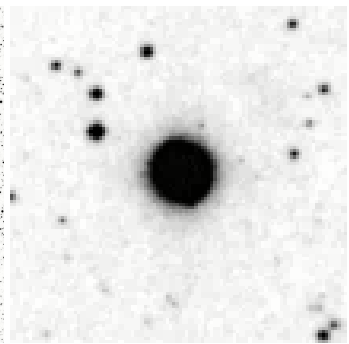
NGC7662 P.N. 3.0'
