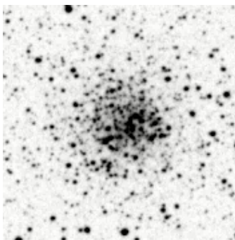
NGC6712 G.C. 5.0'
