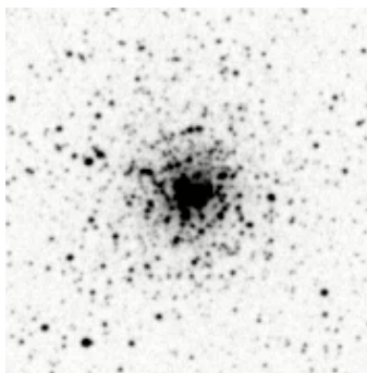
NGC6293 G.C. 5.0'
