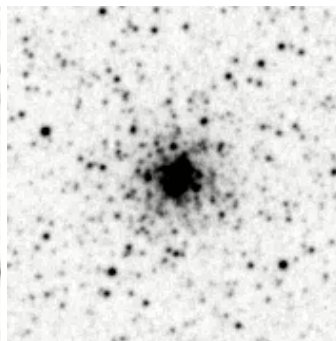
NGC6638 G.C. 5.0'
