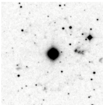
NGC6543 P.N. 7.0'
