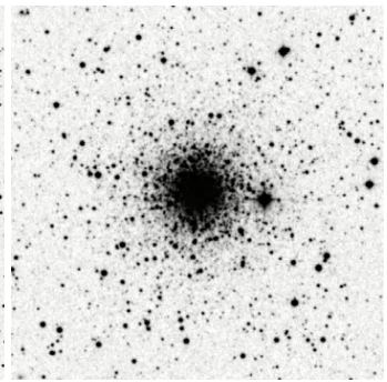
NGC6934 G.C. 10.0'
