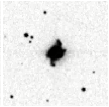
NGC6210 P.N. 5.0'
